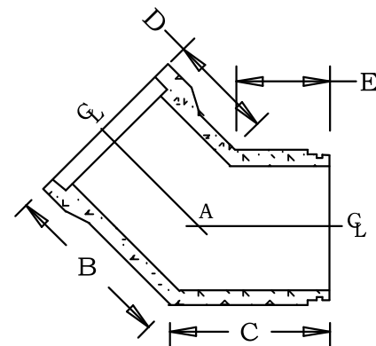
45° Bend
